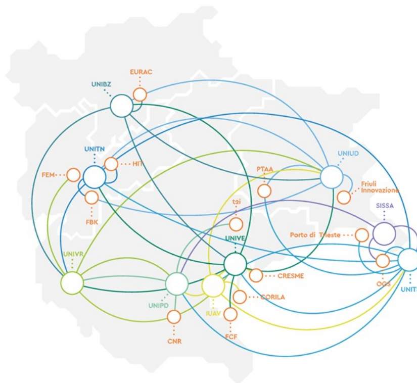
Figura 1 L'ecosistema iNEST
